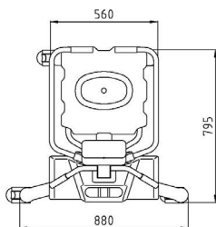
Stollift (mål i mm)
