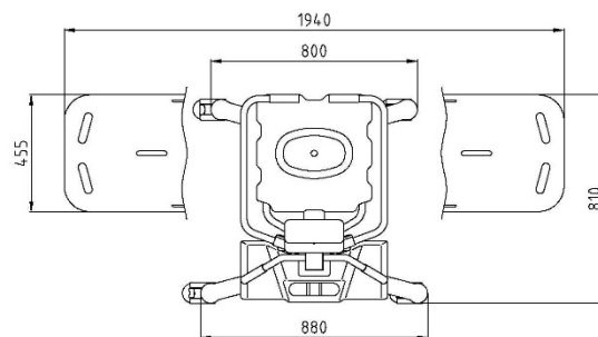
Bruseleje/Kombi-lift (mål i mm)
